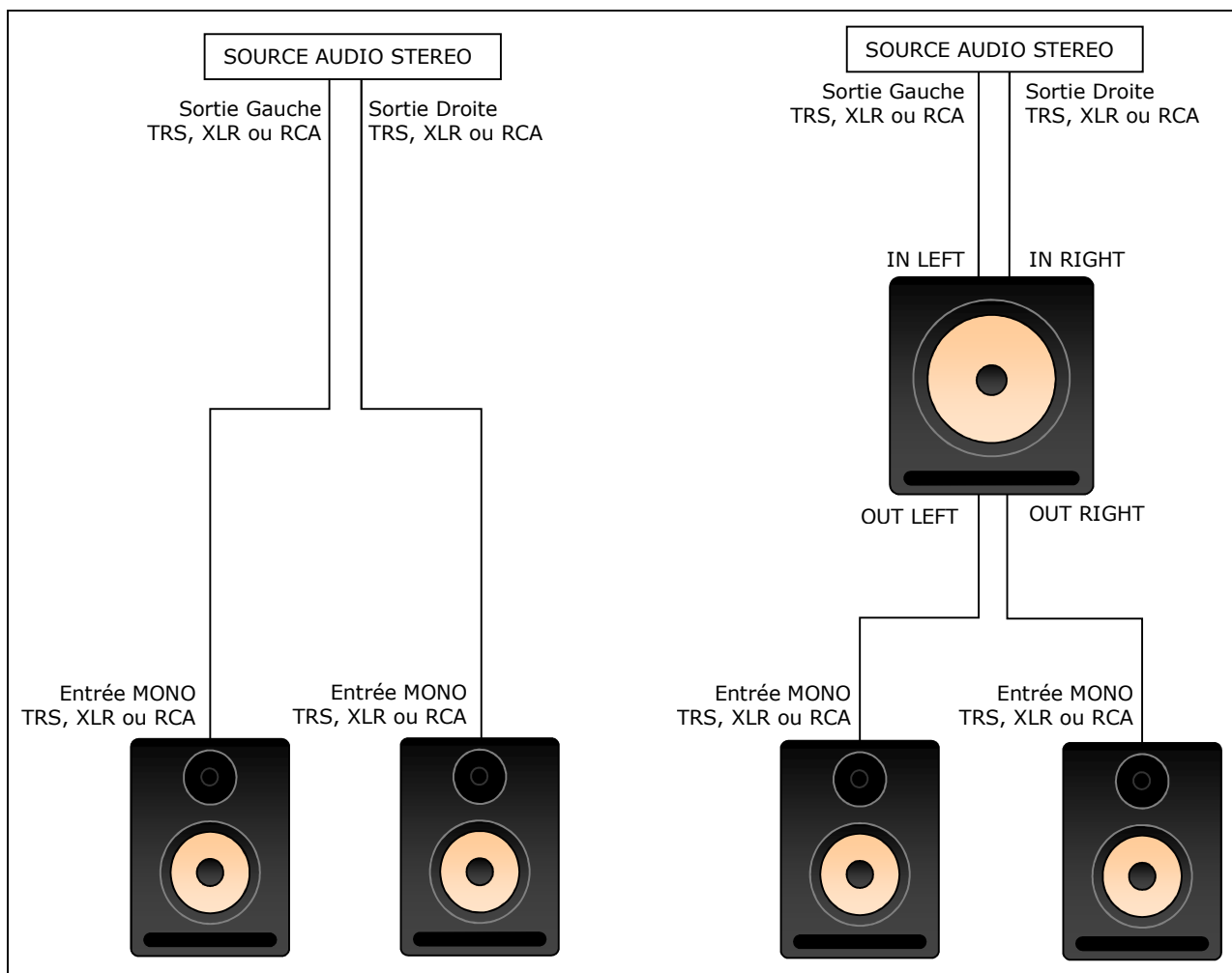
Figure 10 – Branchements stéréo sans/avec caisson
